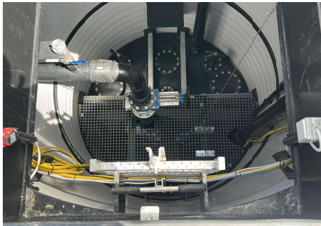
Przepompownia ścieków – tłocznia w Mrokowie.
