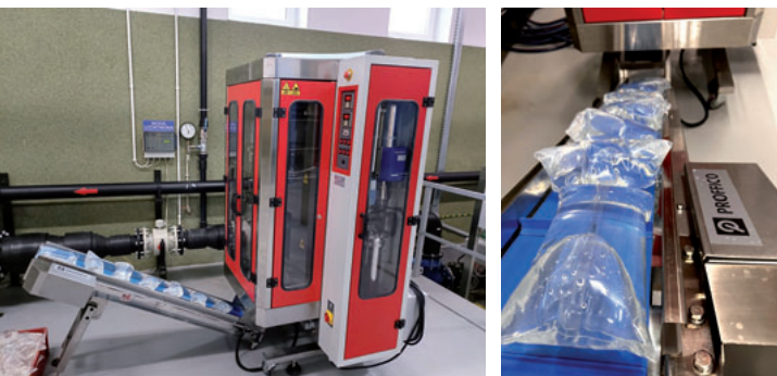
Konfekcjonowanie wody pitnej – paczkowarka
